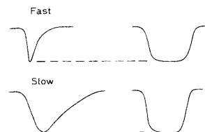
Fig. 14.12. Pulse stretcher function
