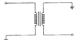
Fig. 14.28. A pulse inverter
